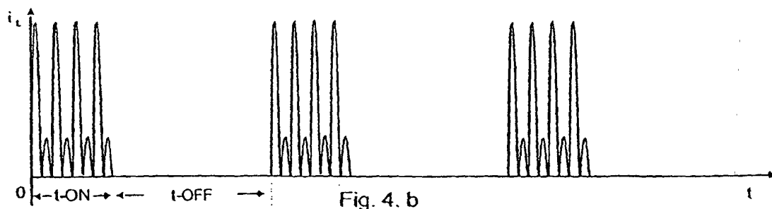
Fig. 4 Low ripple
