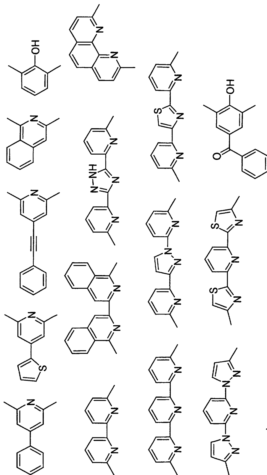
SCHEME 1A
