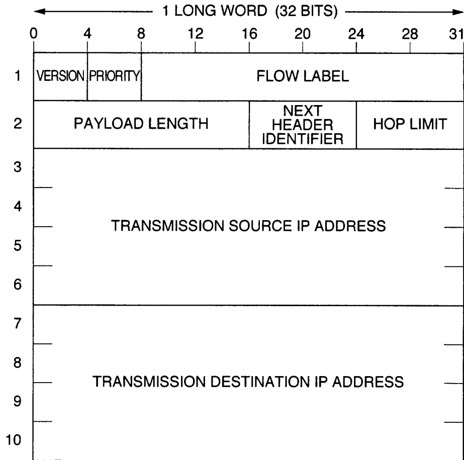
a) IPv6 HEADER FORMAT
