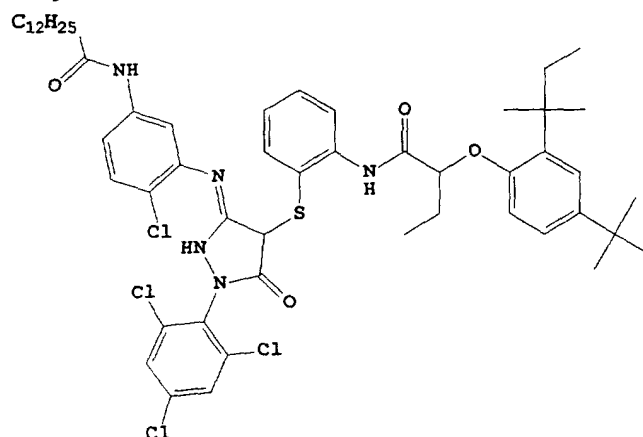
Coupler M1
