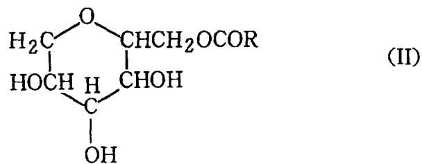
1,5-Sorbitan ester
