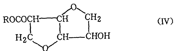
Sorbite ester
