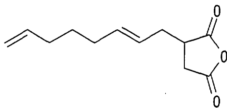
(2,7-octadien-1-yl)succinic anhydride
