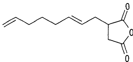
(2,7-octadien-1-yl)succinic anhydride
