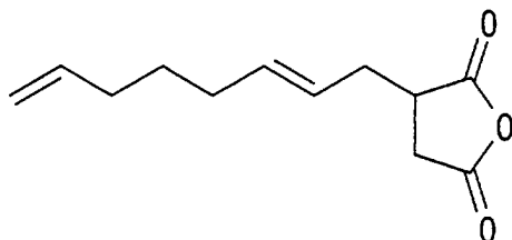
(2,7-octadien-1-yl)succinic anhydride
