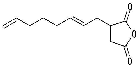
(2,7-octadien-1-yl)succinic anhydride
