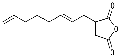
(2,7-octadien-1-yl)succinic anhydride
