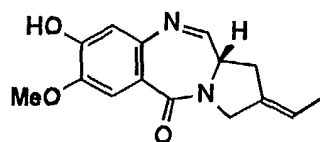
Tomamycin
