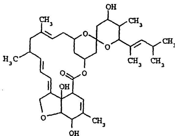
LL-F28249α
