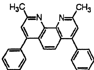
Vasocuproin:
