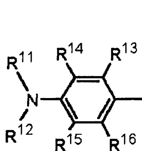
(8)
