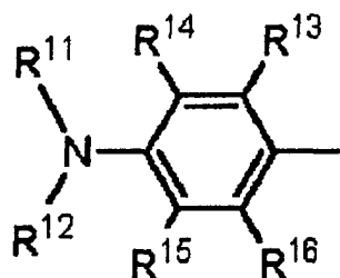
(8)
