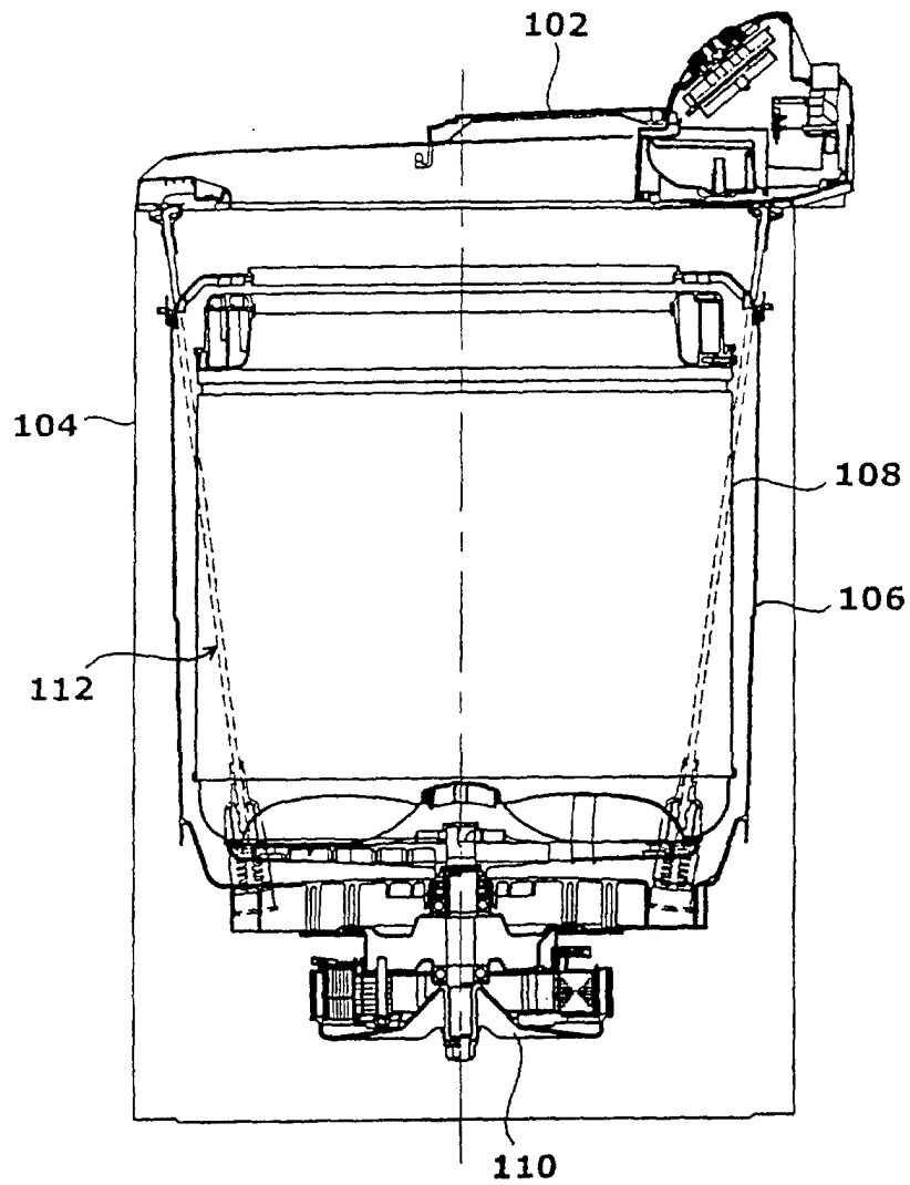
FIG.1(Prior Art)
