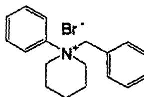
Ammonium salt (4)
