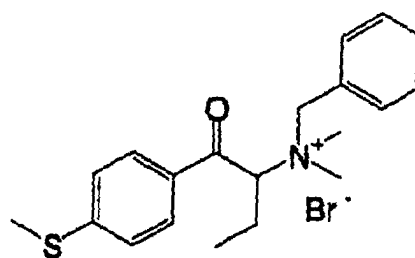
Ammonium salt (2)
