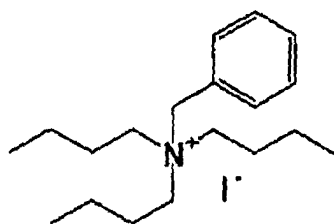
Ammonium salt (1)
