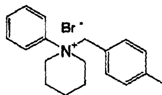
Ammonium salt (6)
