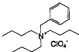
Ammonium salt (7)
