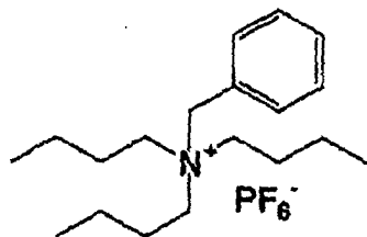
Ammonium salt (3)
