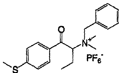
Ammonium salt (5)
