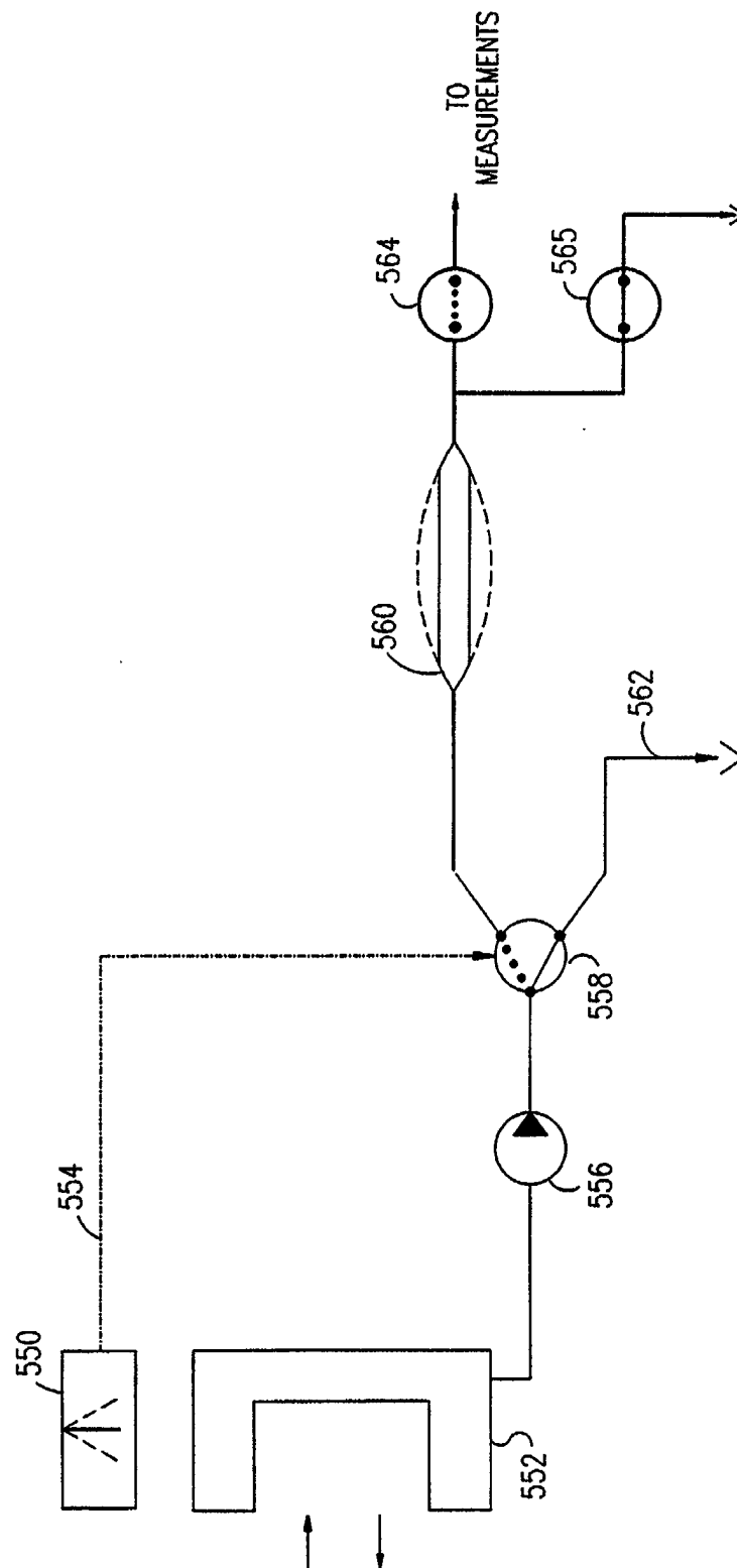
FIG. 35
