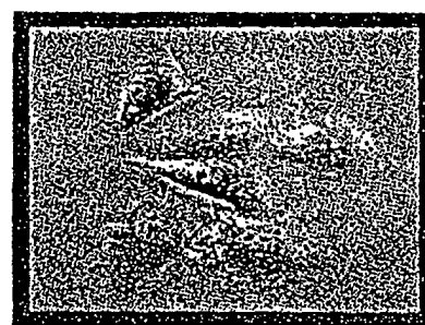
ADN - \text{CaPO}_4
