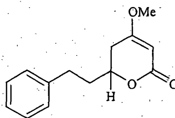
Dihydrokavain
