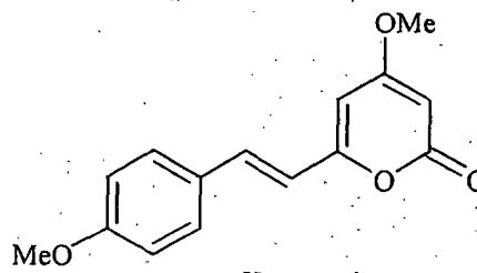
Yangonin
