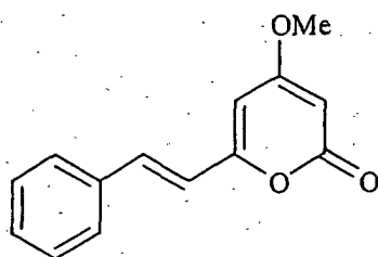
Desmethoxyyangonin
