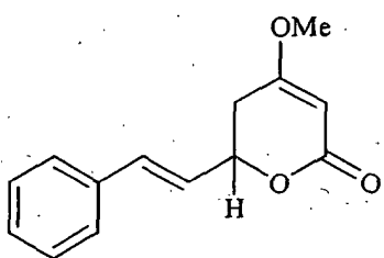
Kavain
