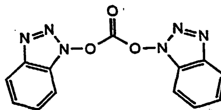
di(1-benzotriazolyl) carbonate
