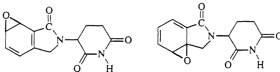
Epoxides of EM 12
