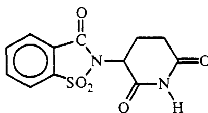
supidimide.
