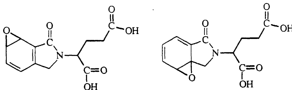
Epoxides of EM 138
