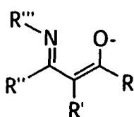
iminoacetones
