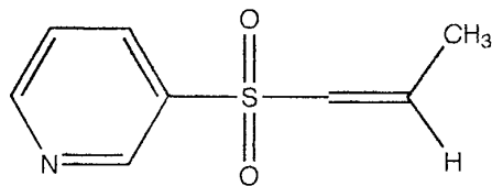
Pyridyl-1-propenyl sulphone
