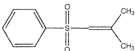
Phenyl-1-isobutenyl sulphone
