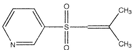
Pyridyl-1-isobutenyl sulphone
