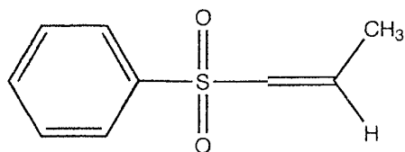
Phenyl-1-propenyl sulphone
