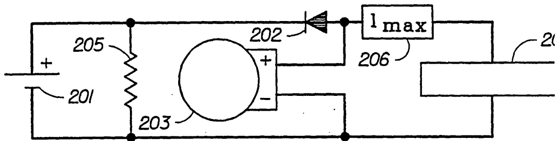
FIG. 14B
