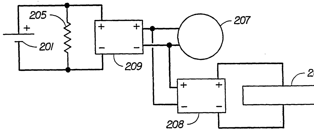
FIG. 14E
