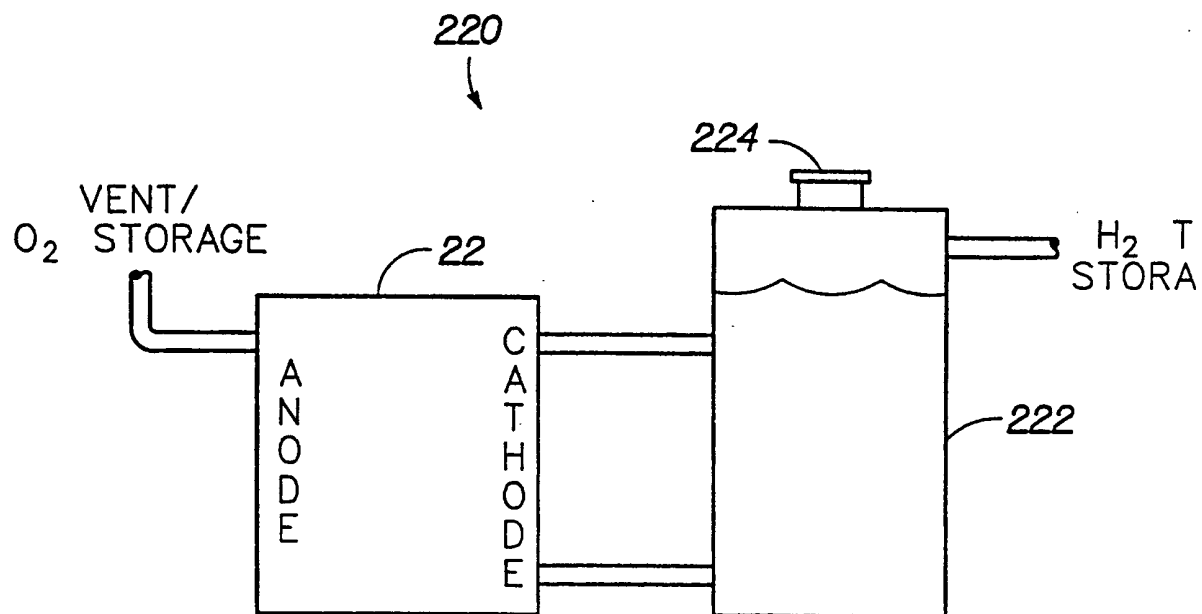
FIG. 35
