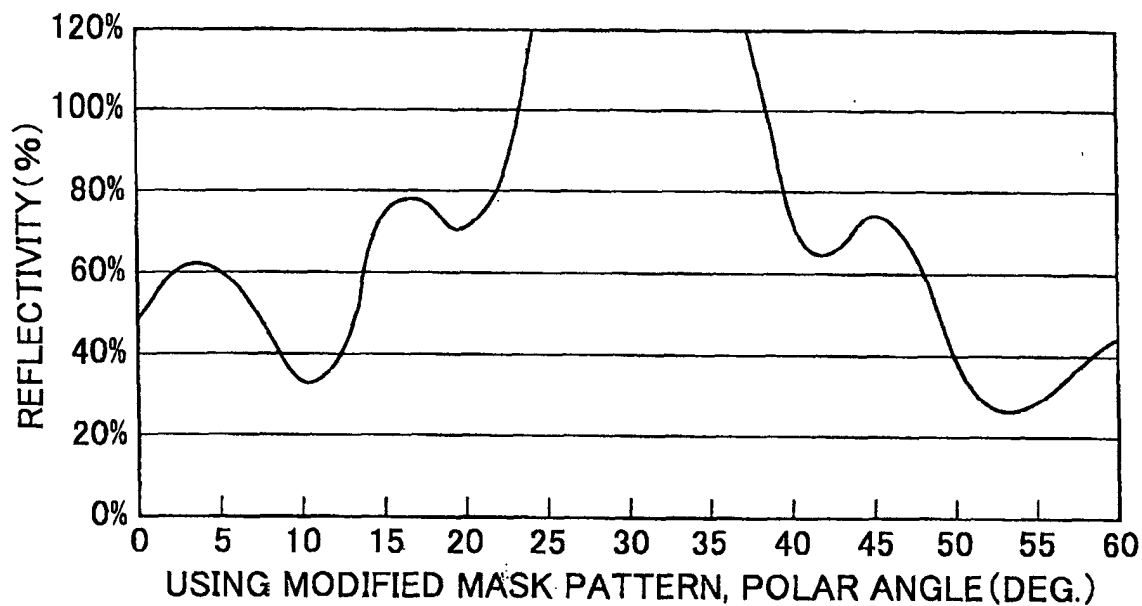
FIG. 16A
