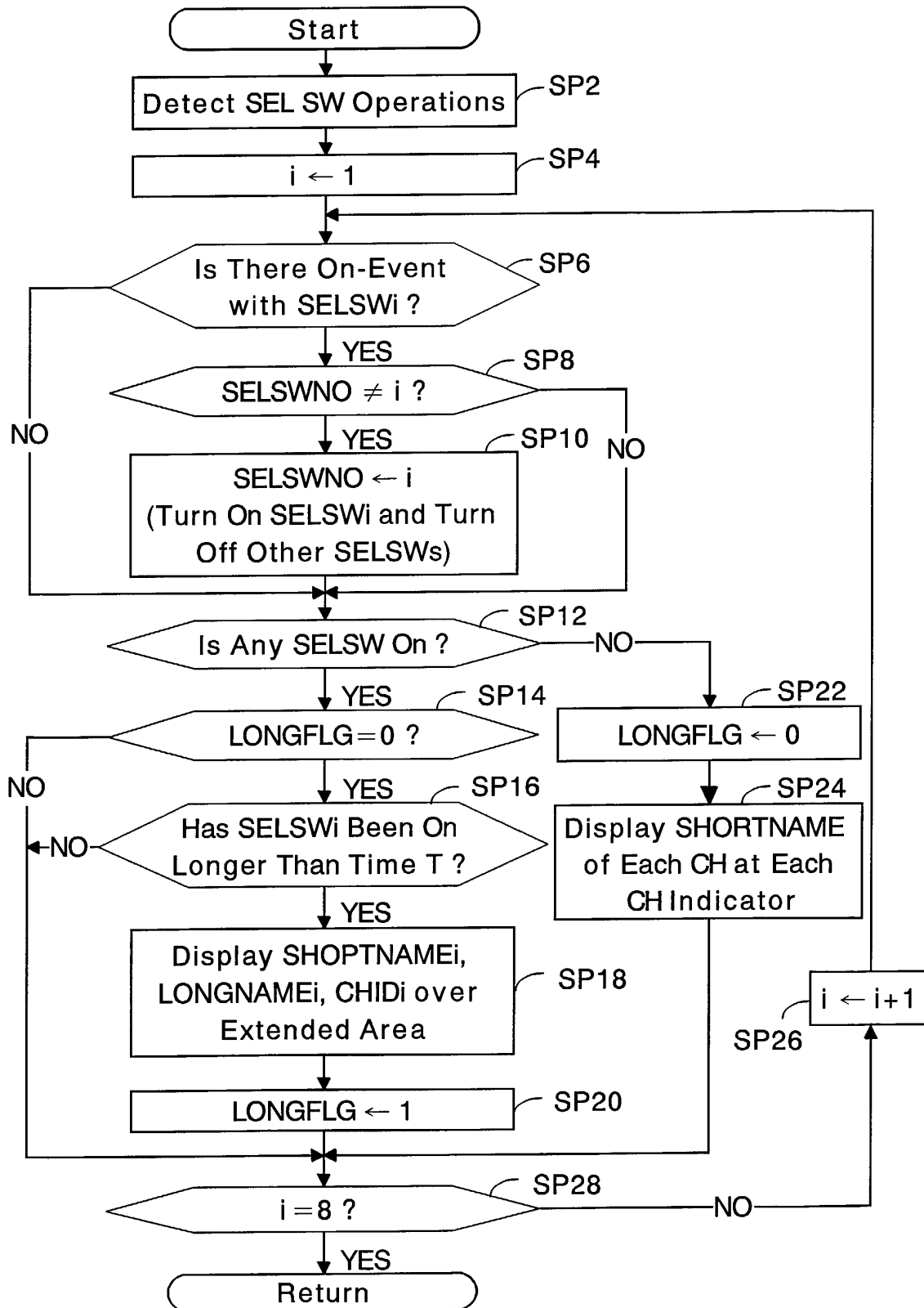
Fig. 5 SEL Control/NAME Display
