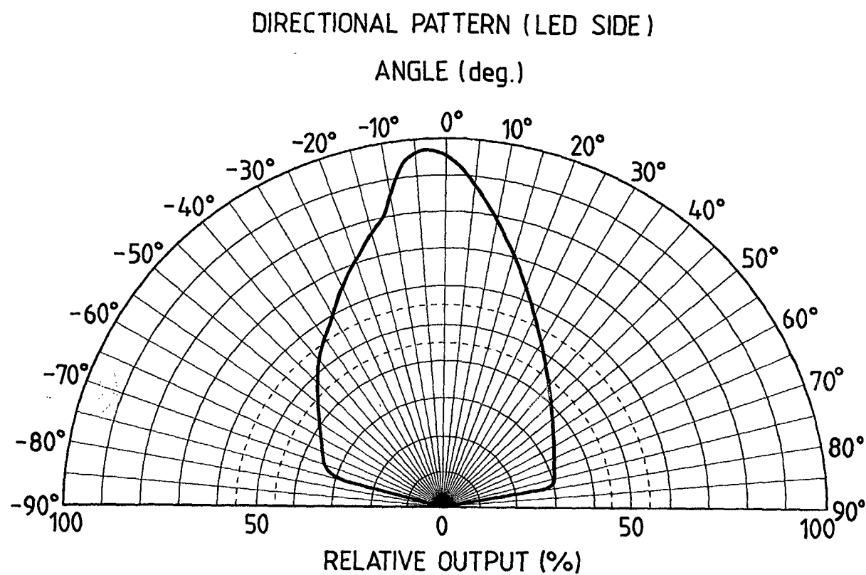
FIG. 14A
