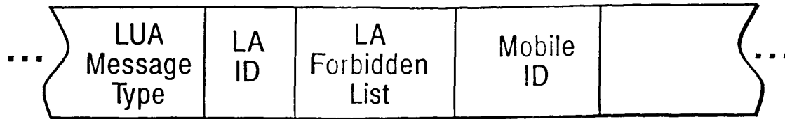
Location Updating Accept (LUA) Message
