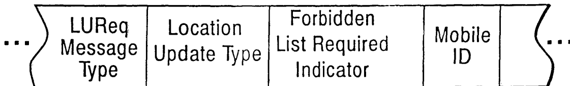
Location Updating Request (LUReq) Message
