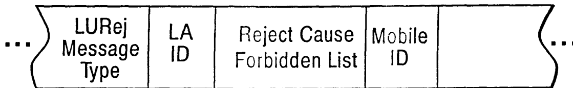
Location Updating Reject (LURej) Message
