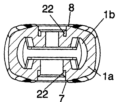
Fig. 6 B-B
