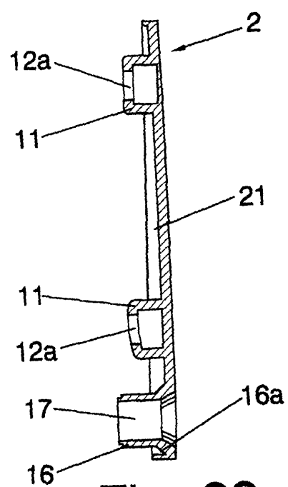
Fig. 22 H-H
