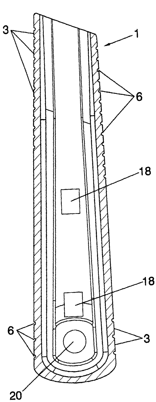
Fig. 8 D-D
