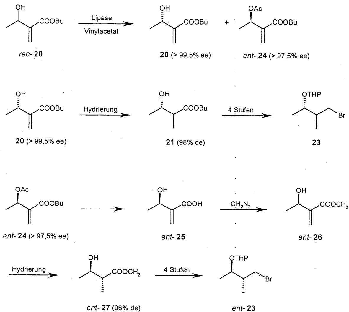
Schema 5
