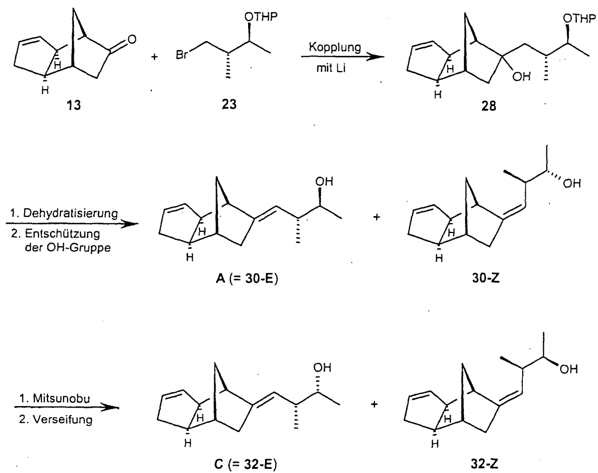
Schema 8
