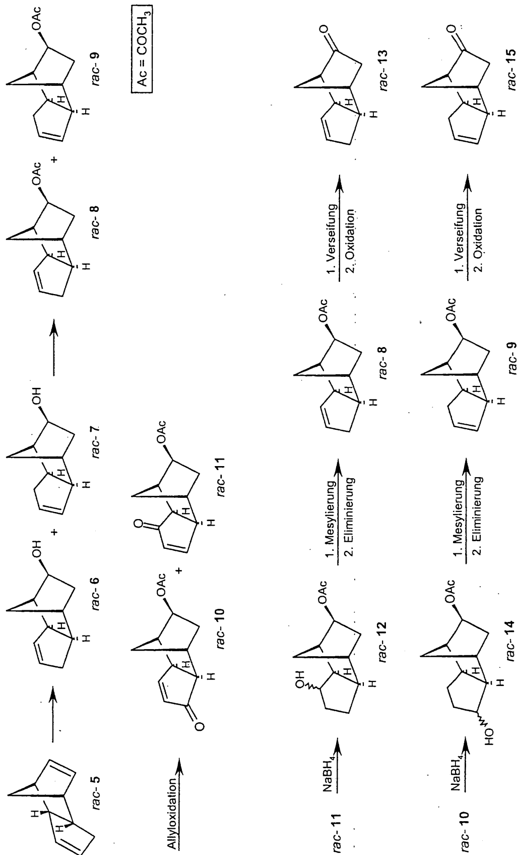
Schema 1
