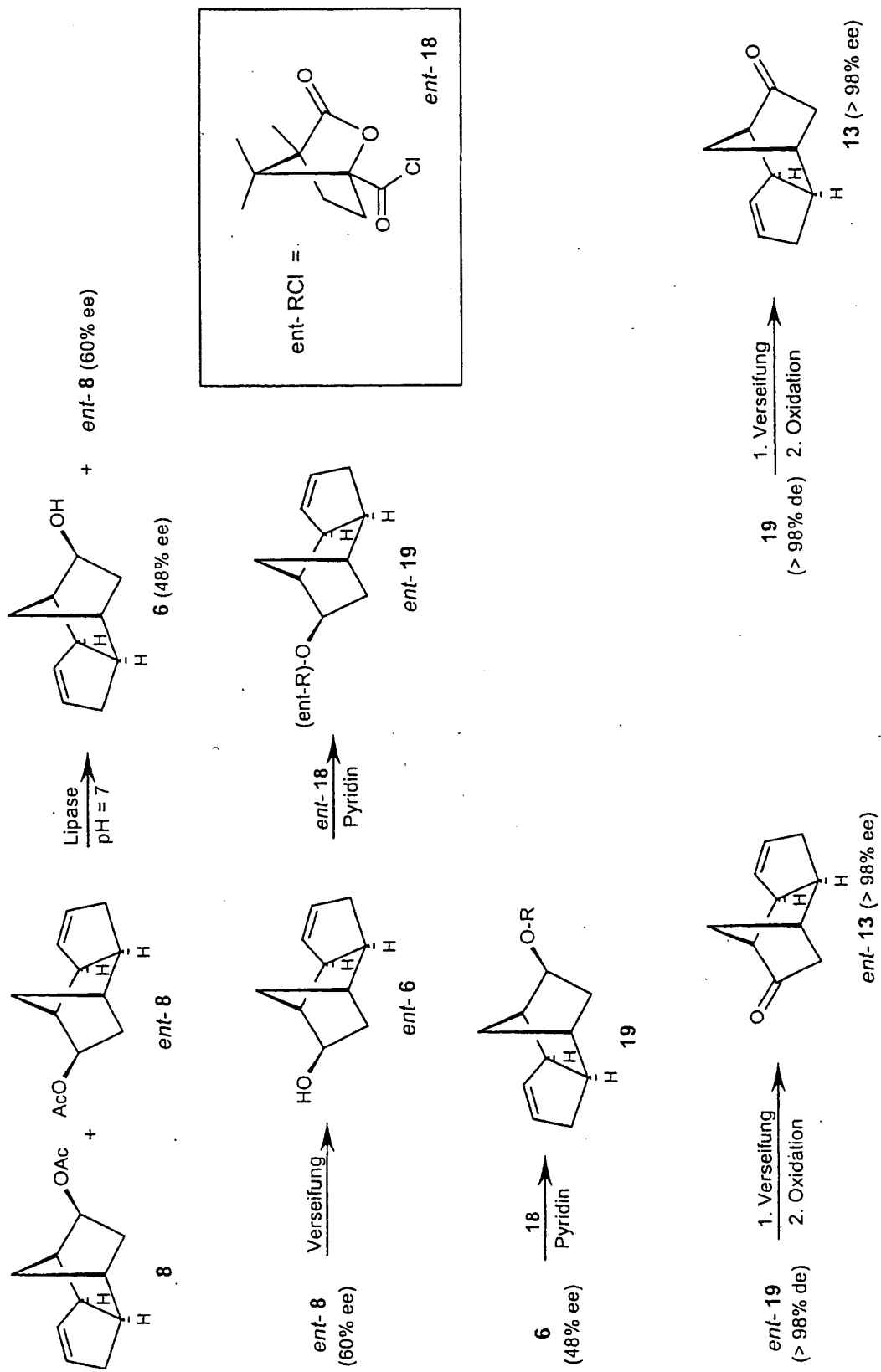
Schema 3
