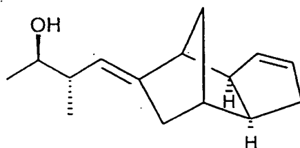
ent-A
