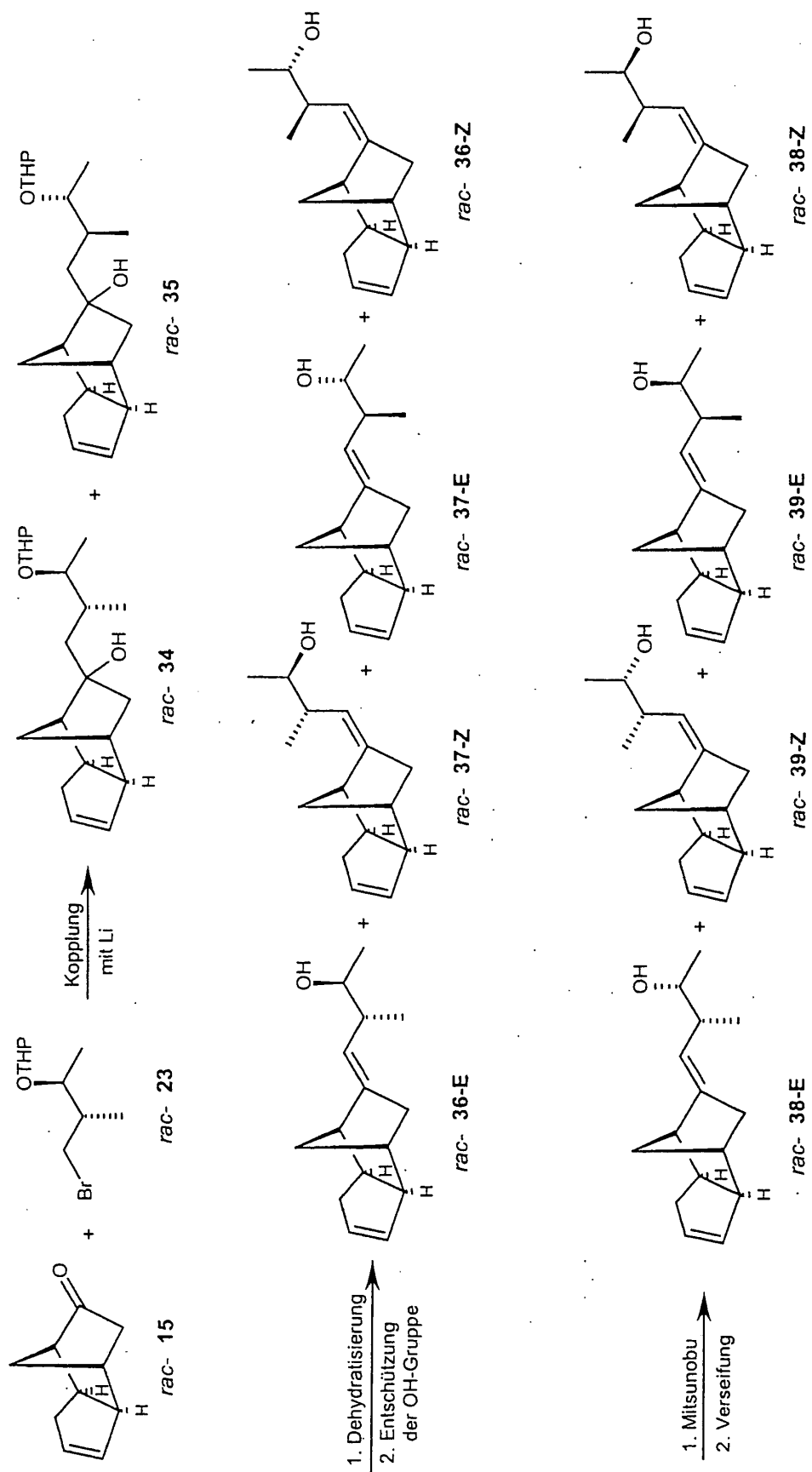
Schema 7
