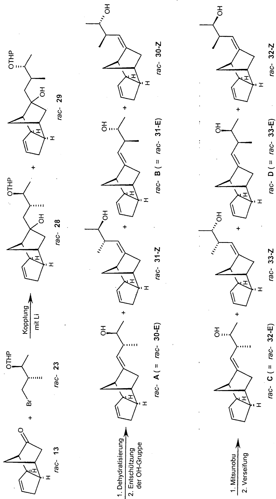
Schema 6
