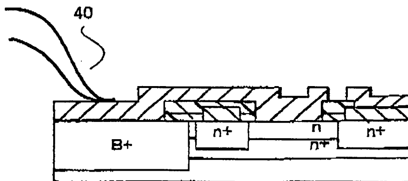
FIG.7E
