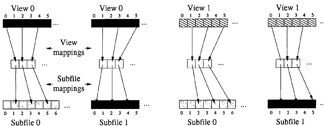
(d) View and subfile mapping
