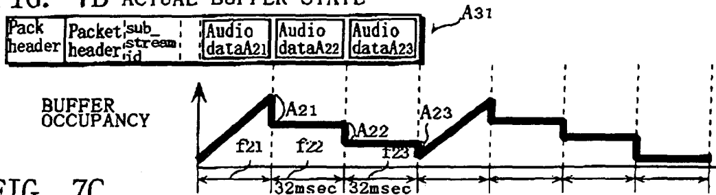
FIG. 7B ACTUAL BUFFER STATE
