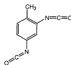
Tolylene 2,4 disioscyanate
