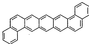
1,2;8,9-dibenzopentacene
