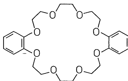
Dibenzo-24-crown 8-ether
