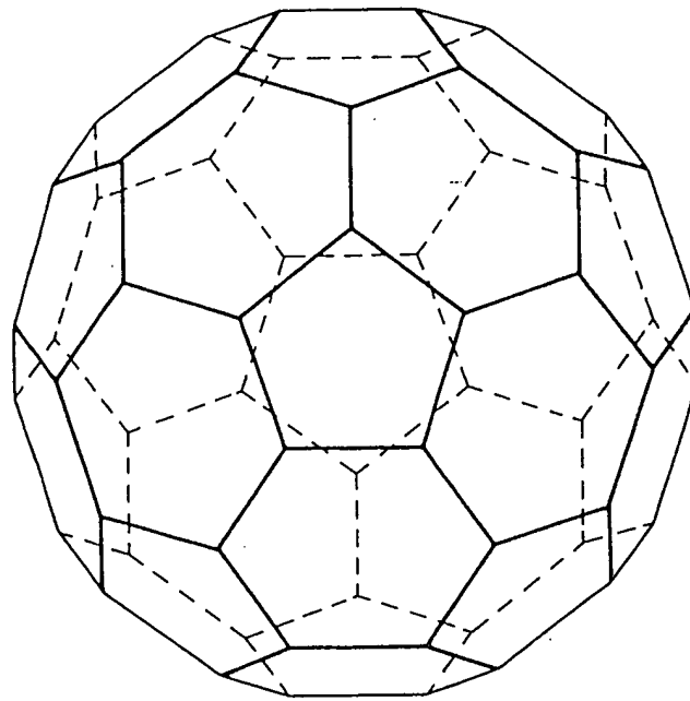
C 60
