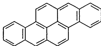
Dibenzo(b,def) chrysene
