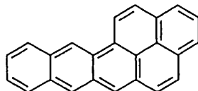
Naphtho(2,3-a)pyrene
