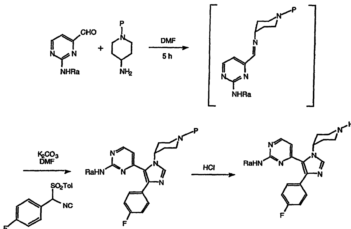
SCHEME VI
