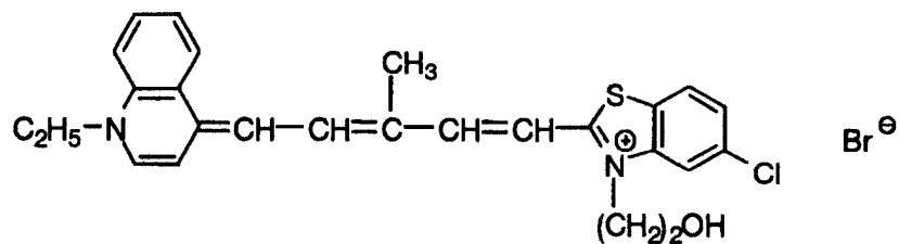
VIa-10
