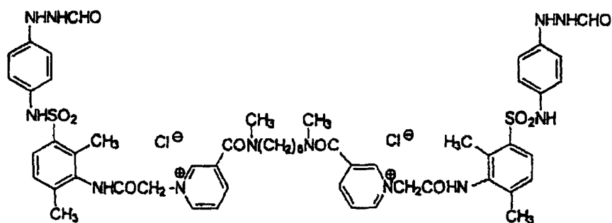
(D-83)
