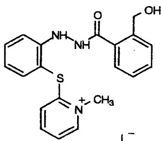
(D-117)
