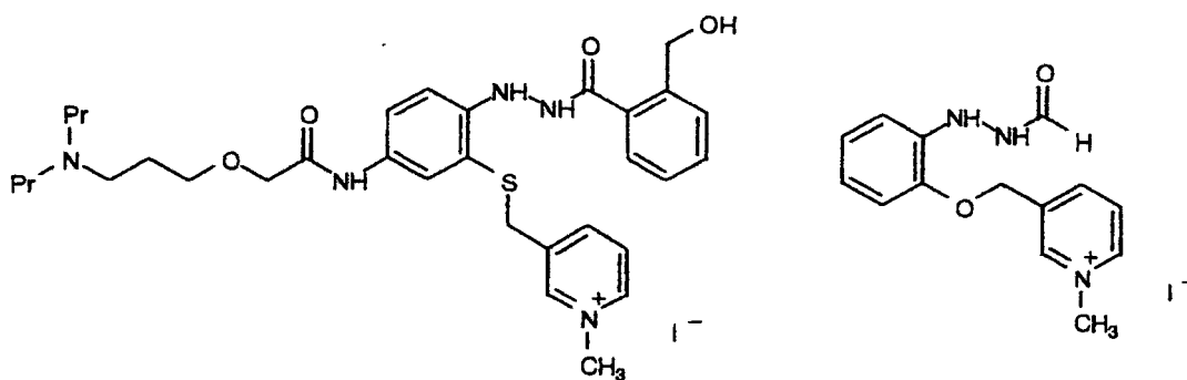
(D-125)
