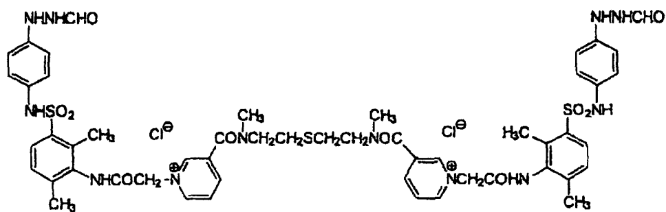
(D-84)
