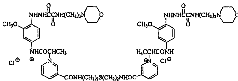
(D-105)
