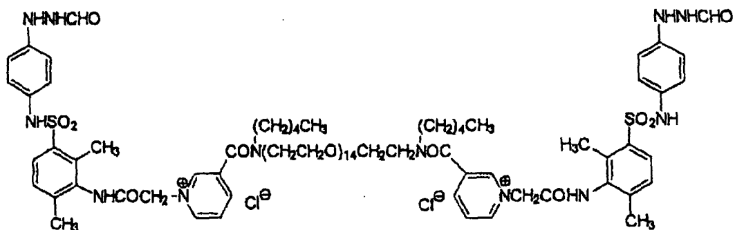
(D-86)
