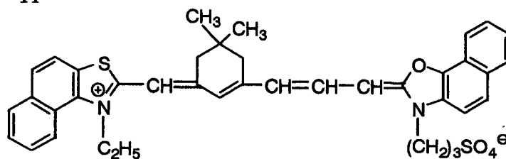
VIb-11
