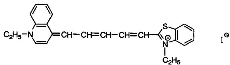
VIa-3
