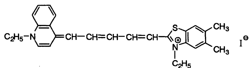
VIa-3
