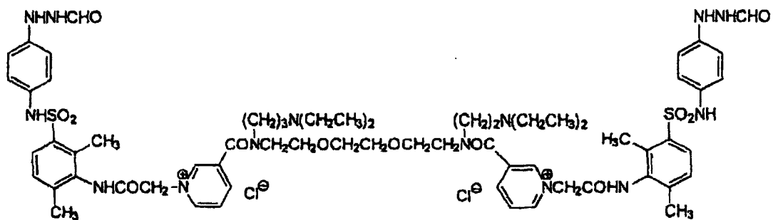
(D-85)
