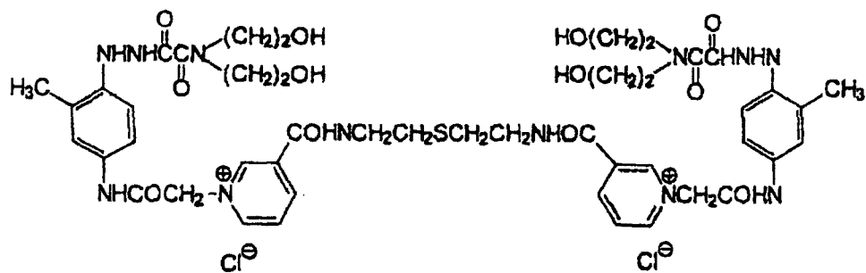
(D-78)
