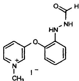
(D-127)
