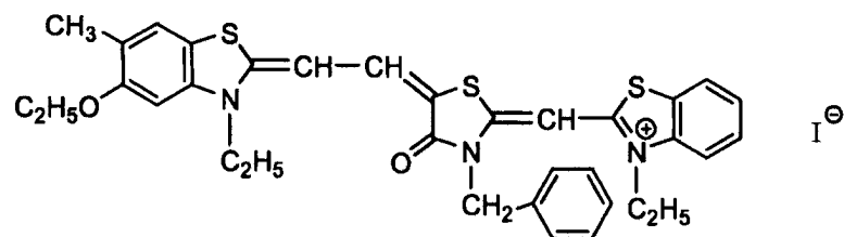
V - 37
