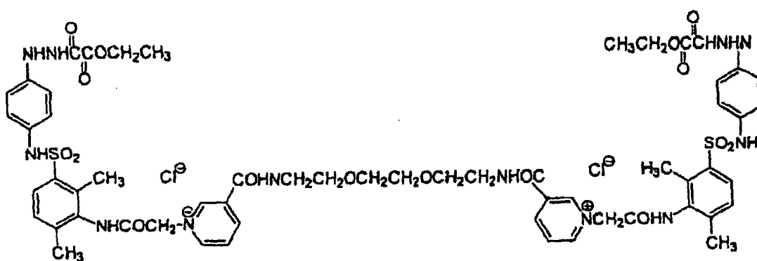
(D-76)
