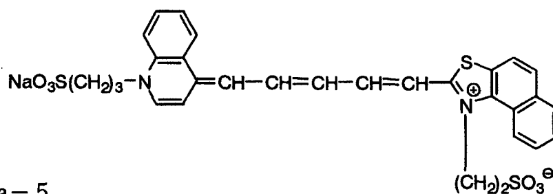
VIa-4
