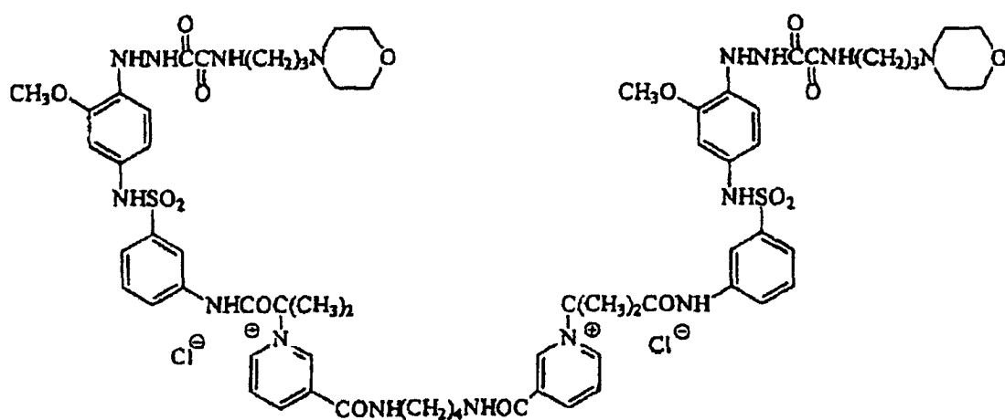
(D-104)
