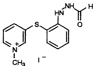
(D-119)
