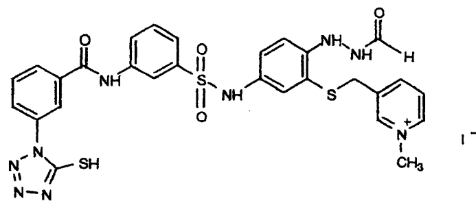
(D-114)
