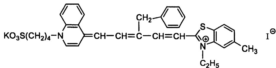
VIa-13
