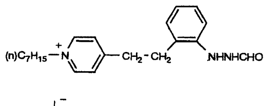
(D-128)
