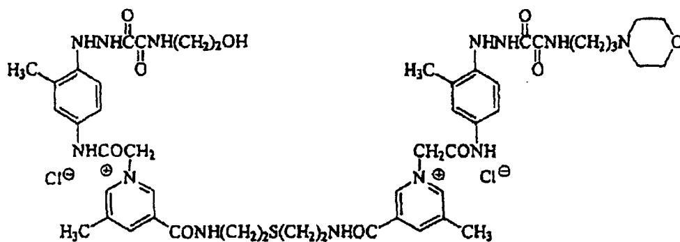
(D-103)
