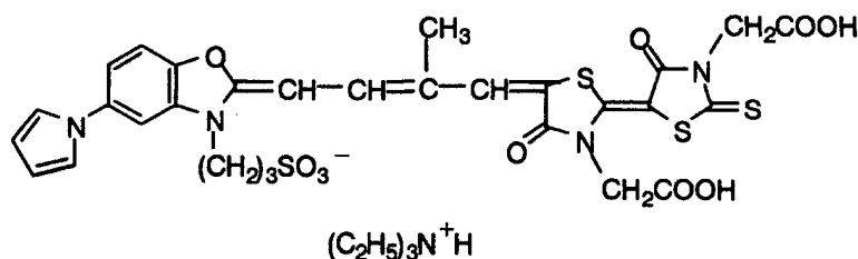
II-1
