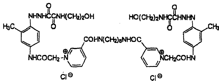
(D-77)
