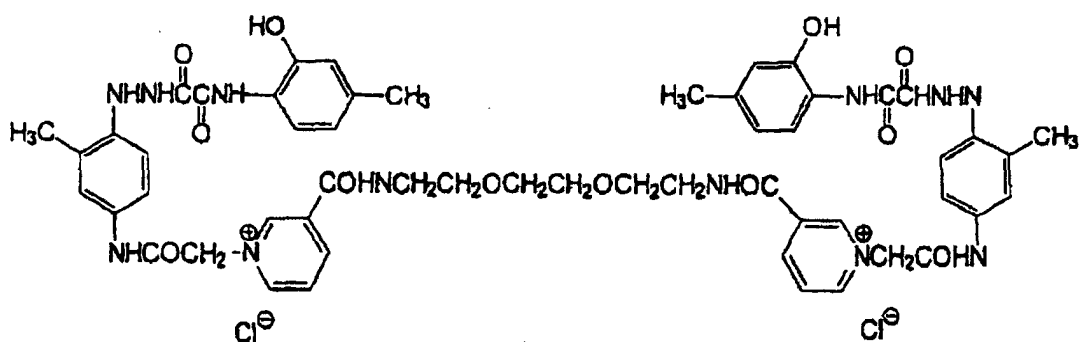
(D-79)
