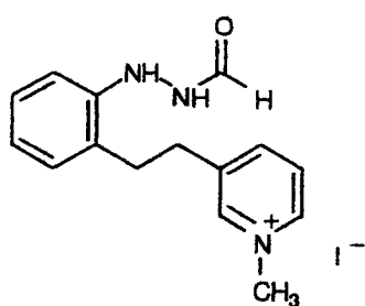
(D-115)
