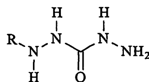
carbazine
