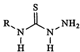
thiosemicarbazide
