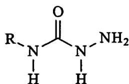
semicarbazide
