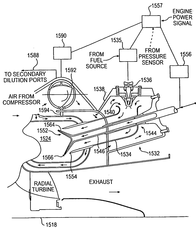
FIG. 18A
