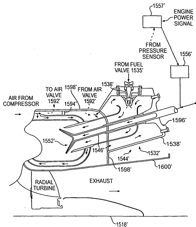
FIG. 18C
