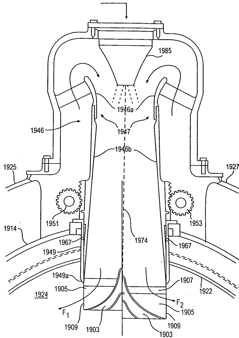
FIG. 19C
