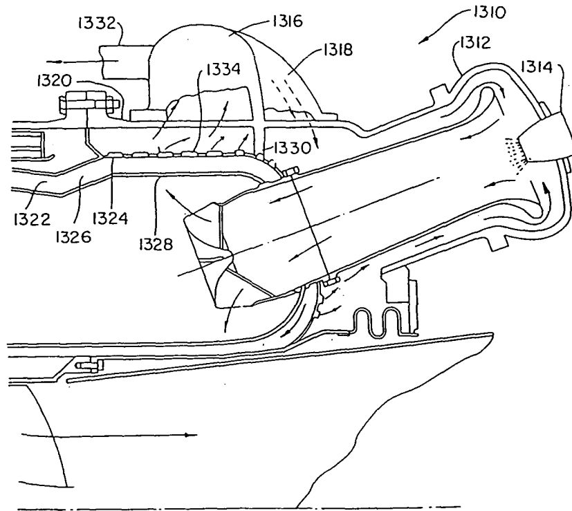
FIG. 15A
