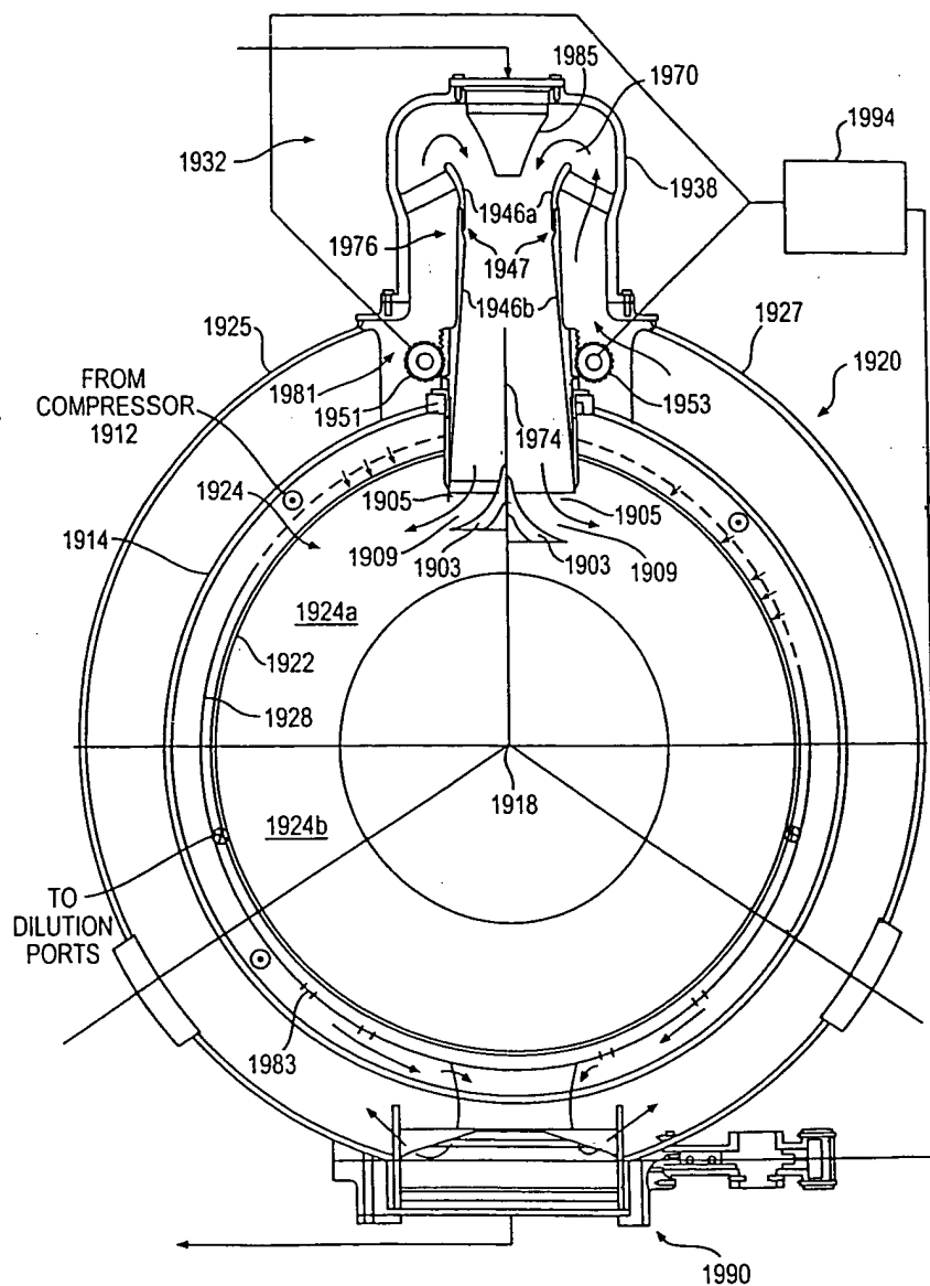
FIG. 19B
