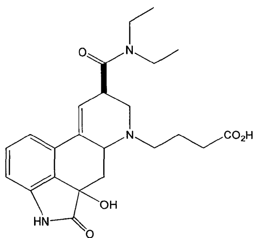
Haptent B
