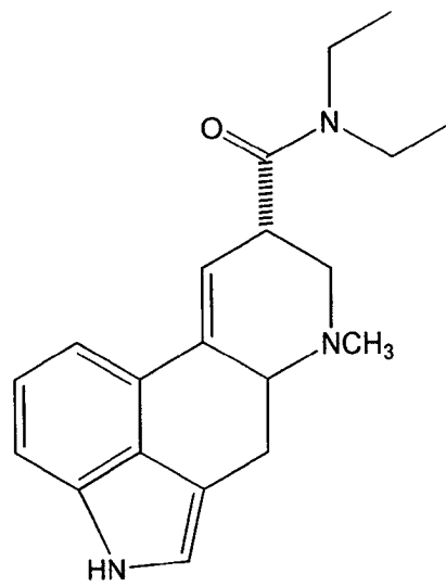
iso-LSD 2
