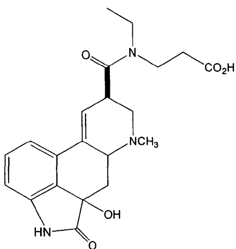
Haptent A
