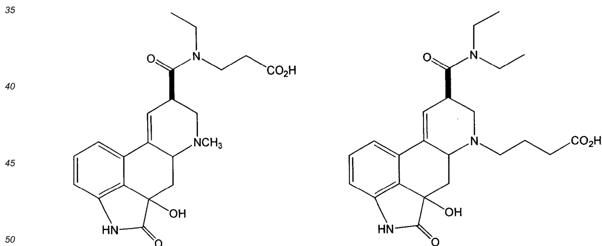
Hapten A
