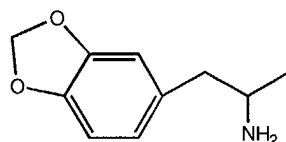
3 MDA
