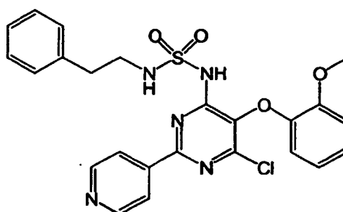
LC-MS: t_R : 4.90; [M+H]^+ : 512.18
