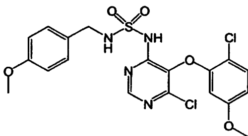
LC-MS: t_R : 4.93; [M+H]^+ : 484.95
