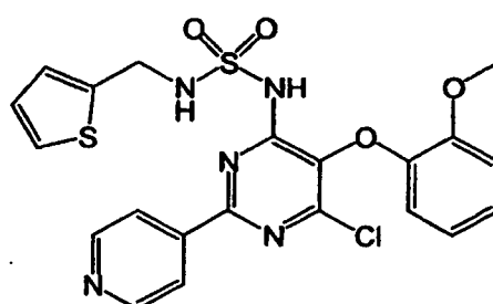
LC-MS: t_R : 4.57; [M+H]^+ : 504.06
