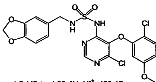
LC-MS: t_R : 4.89; [M+H]^+ : 499.17
