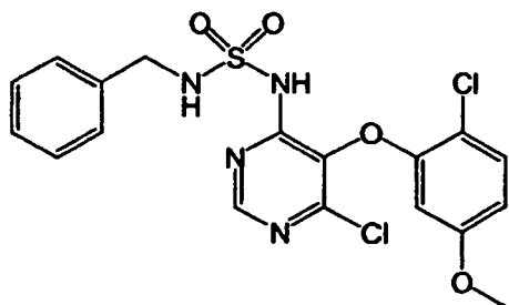
LC-MS: t_R : 5.13; [M+H]^+ : 456.91
