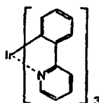
Ir(ppy) 3
