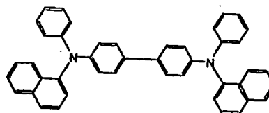
\alpha -NPD
