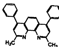
BCP
