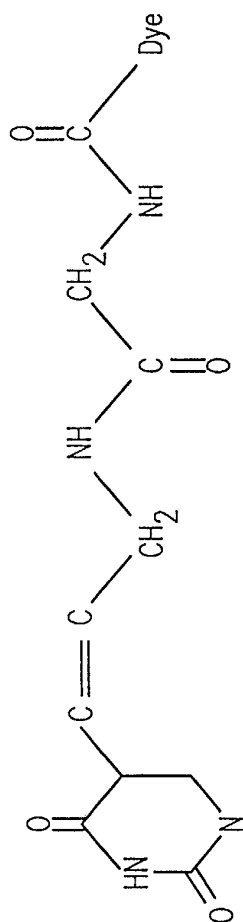
Diglycinyllinker
