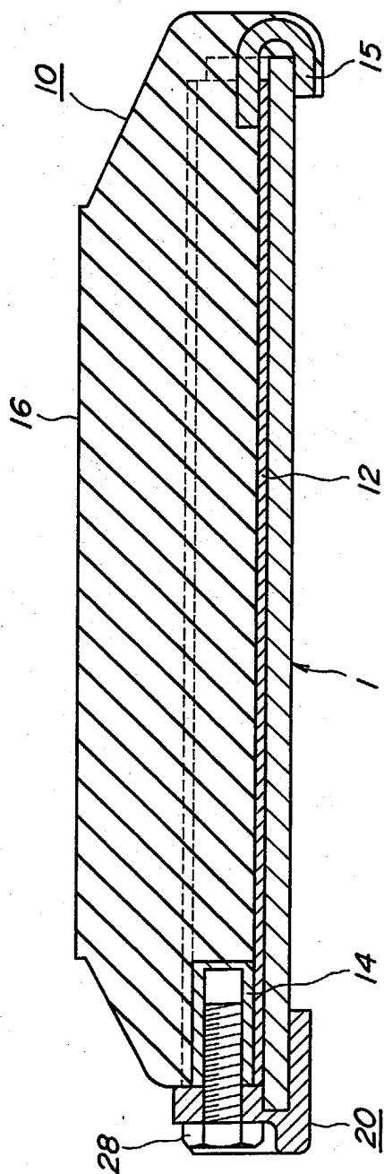
FIG. 12
