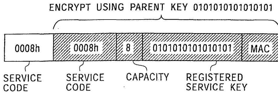
FIG. 17B
