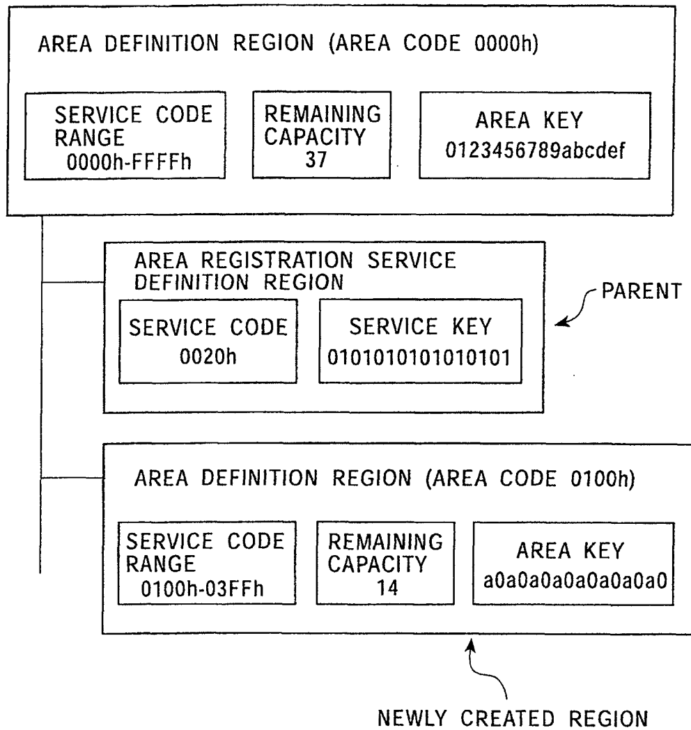
FIG. 16A
