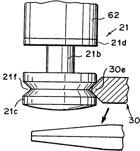
FIG. 16A
