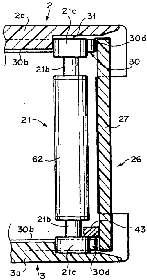
FIG. 23
