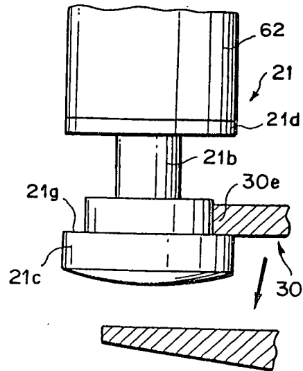
FIG. 16D
