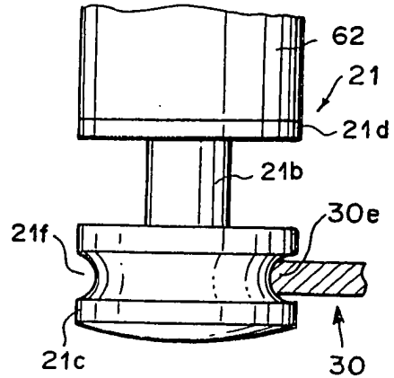
FIG. 16B
