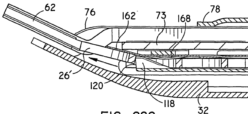
FIG. 22C
