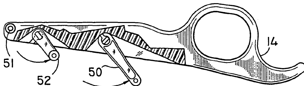
FIG. 18C
