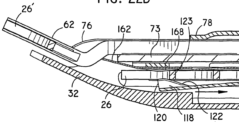
FIG. 22E
