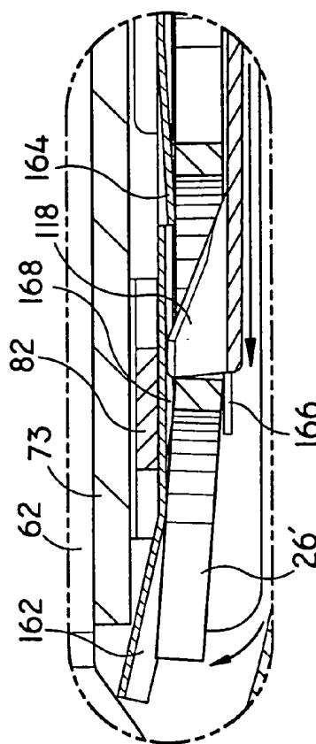
FIG. 22B
