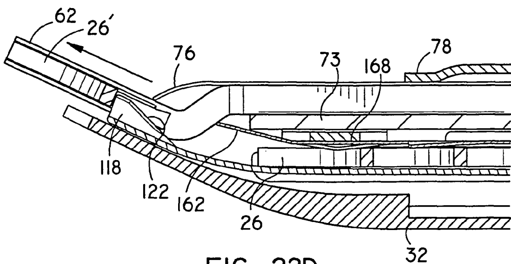
FIG. 22D
