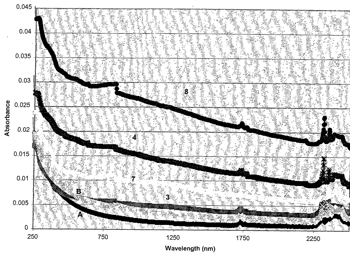
IR - UV - Visible Spectrum
