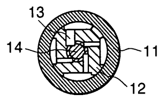
A-A SECTION
