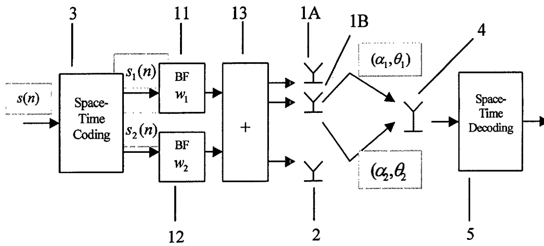
Figure4: Prior Art
