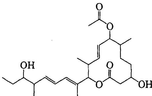
11107BJ
