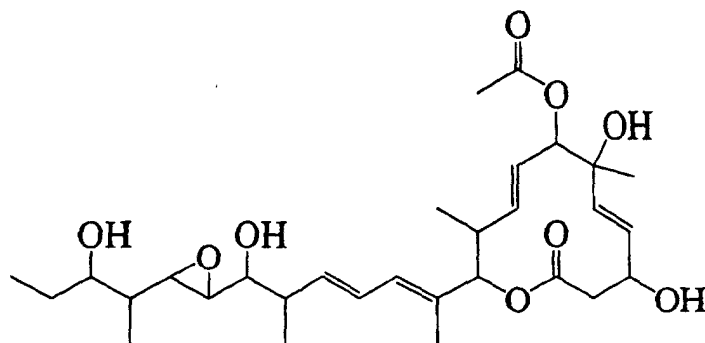
11107AX
