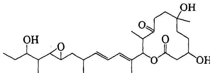
11107V
