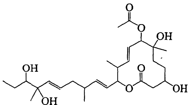
11107BC
