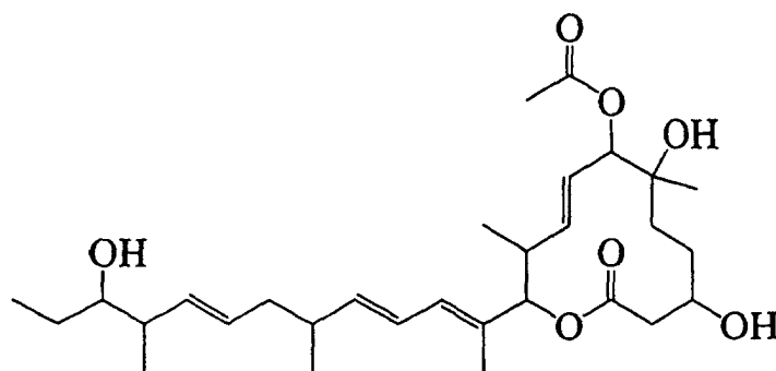
11107BI
