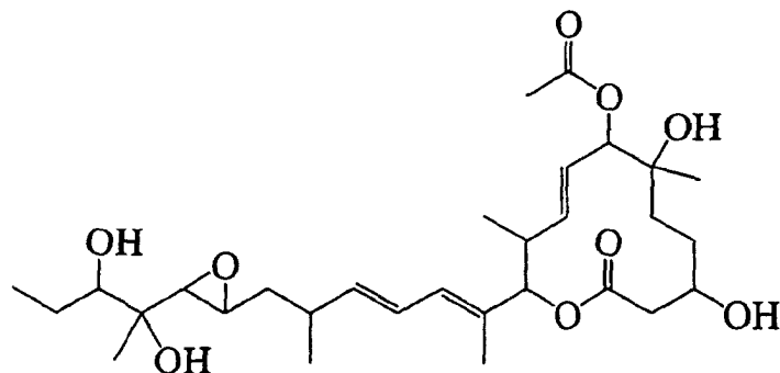
11107E
