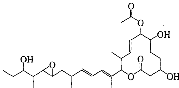
11107AEa
