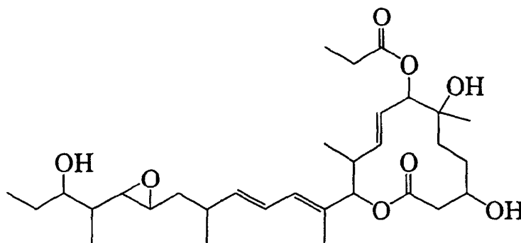
11107I
