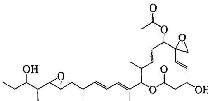
11107AN
