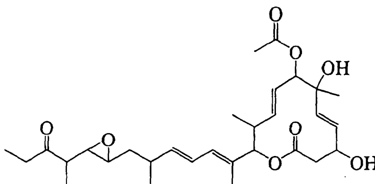
11107AL
