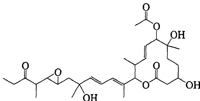
11107AV
