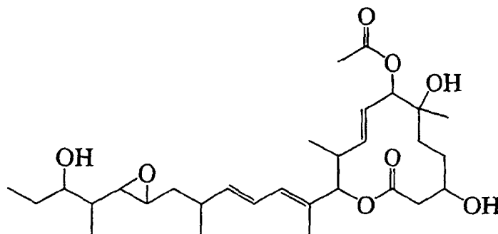
11107B
