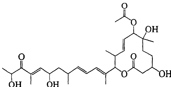
11107Q
