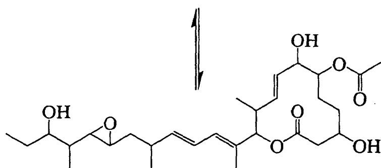
11107AEb
