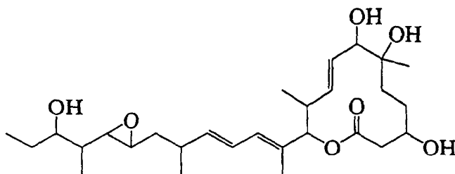
11107A
