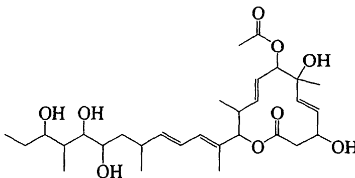
11107BA
