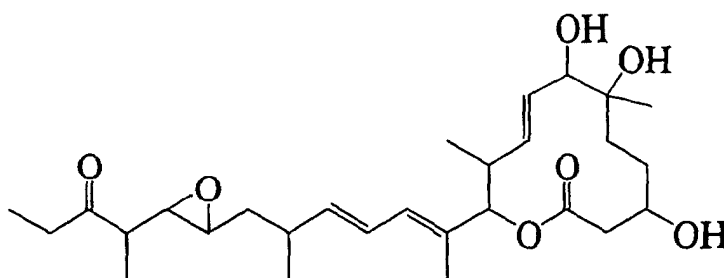
11107AC
