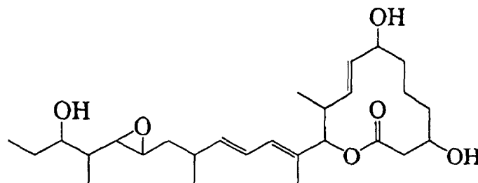
11107AK
