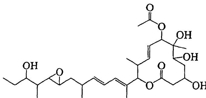
11107K
