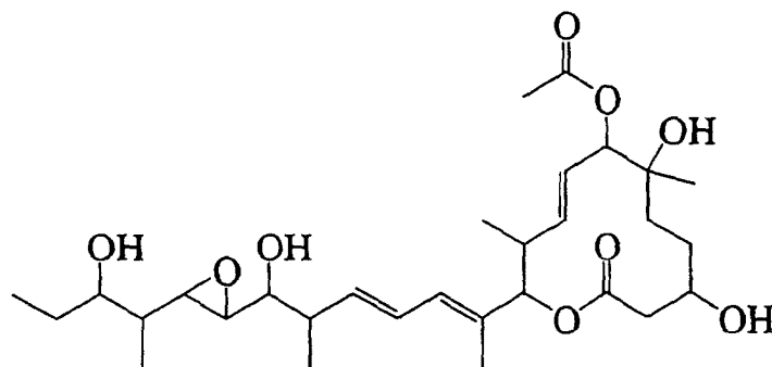
11107P
