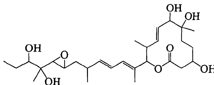
11107G
