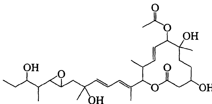
11107D
