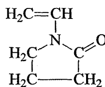
2-vinylpyrrolidone
