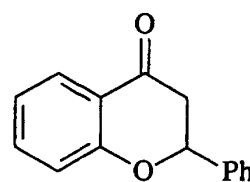
Racemic form (d)
