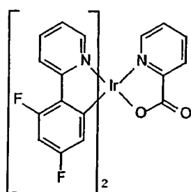
Ir(pic)
