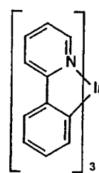
Ir(ppy) 3
